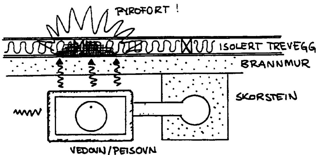
Tegning: Selvantennning i vegg bak brannmur
